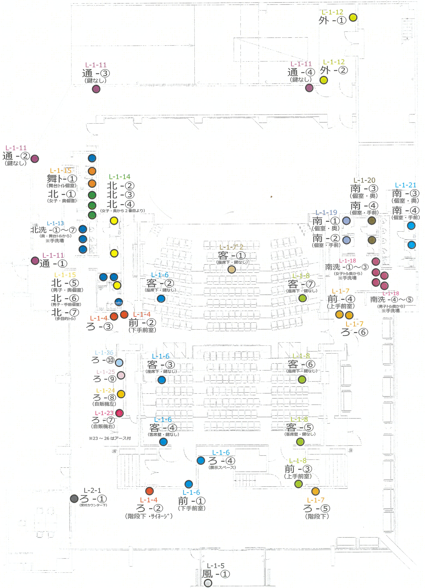
木曽川文化会館 ホール棟平行コンセント回路図
